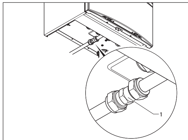
Afb. 5.1 Gasaansluiting
