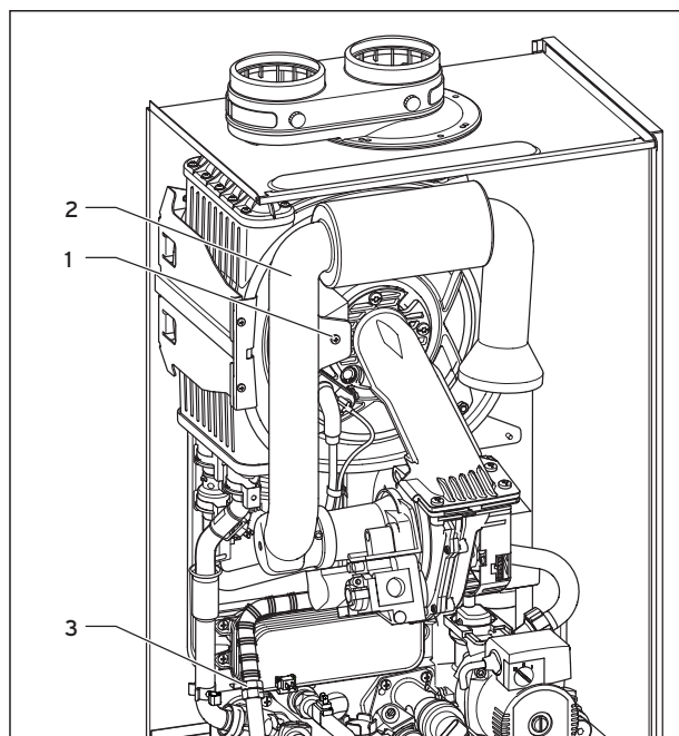
Afb. 8.1 Luchtaanzuigbuis demonteren
