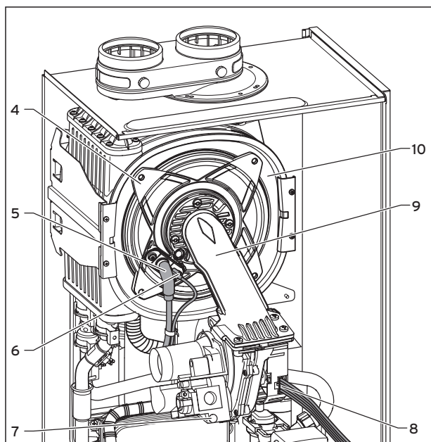
Afb. 8.2 Brander-ventilator-gasblok demonteren
