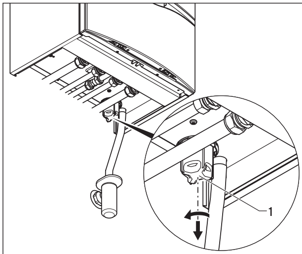
Afb. 6.3 Condenswatersifon vullen
