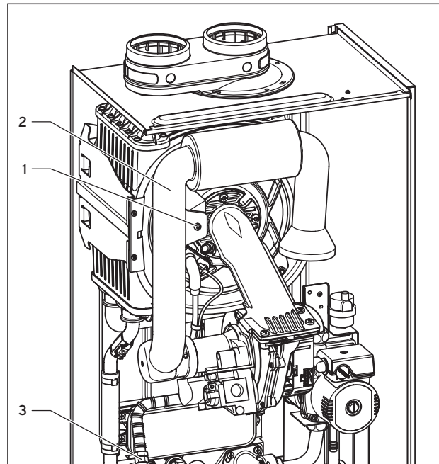
Afb. 8.7 Luchtaanzuigbuis demonteren
