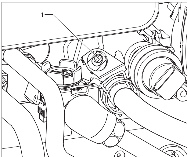
Afb. 7.3 Bypass-ventiel instellen
