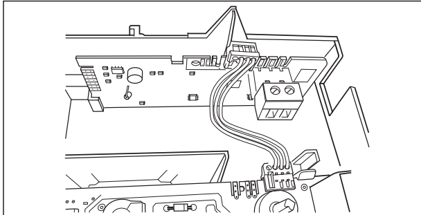
Afb. 5.9 Aansluiting Opentherm-Modul
