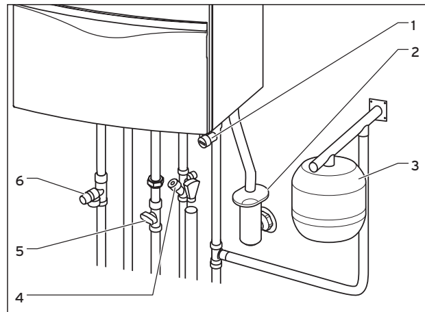
Afb. 5.4 Aanbevolen toestelaansluiting
