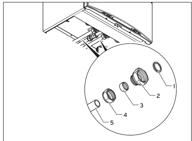
Afb. 5.2 Koud- en warmwateraansluiting monteren
