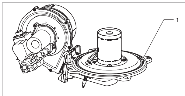
Afb. 8.5 Pakkingen vervangen
