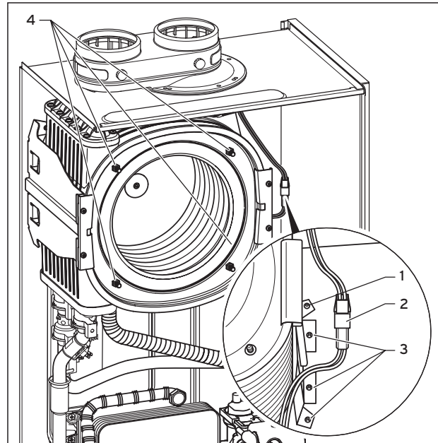
Afb. 10.5 Houder van de primaire warmtewisselaar
