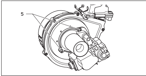
Afb. 10.3 Schroefverbinding gasblok/ventilator
