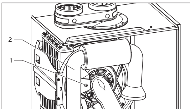
Afb. 8.10 Demontage van de zeef in de koudwateringang.
