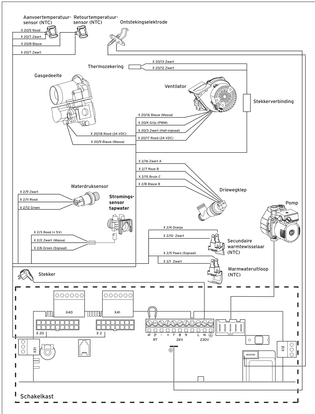
Afb. 5.11 Aansluitschema hrSOLIDE plus
