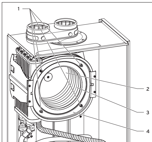
Afb. 8.3 Primaire-warmtewisselaar reinigen
