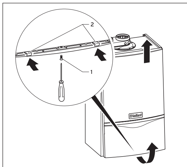
Afb. 4.5 Voorpaneel demonteren
