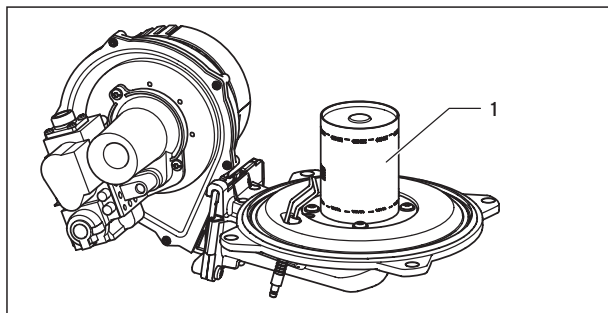
Afb. 8.4 Brander controleren
