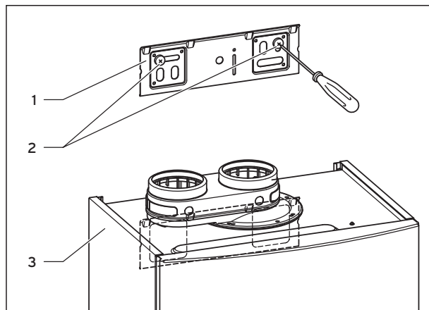
Afb. 4.4 Toestel ophangen
