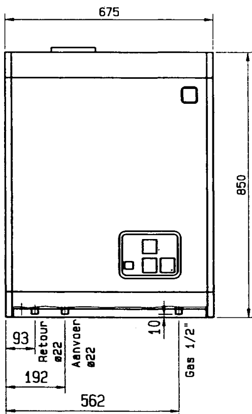
VOORAANZICHT
