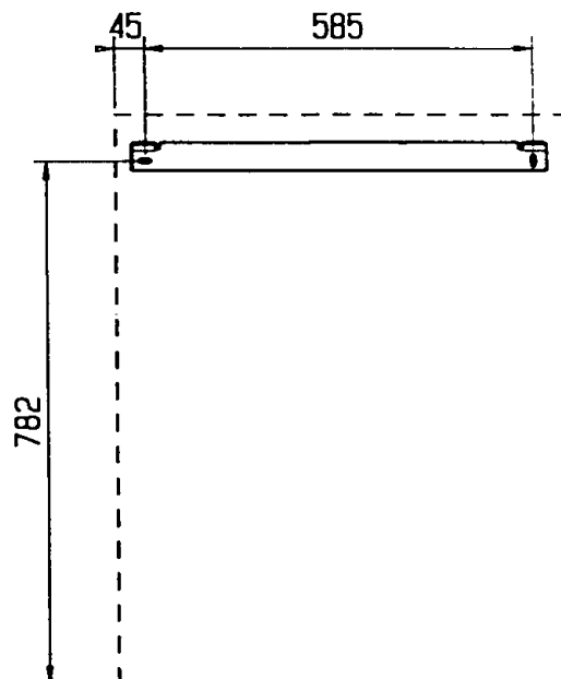
ZIJAANZICHT
