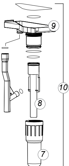
Sifon figuur 13.5.g
