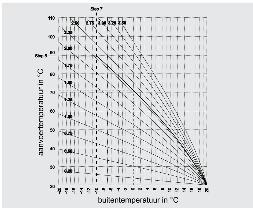
stroomlijnstellingen Parameter Step 6 en 7
